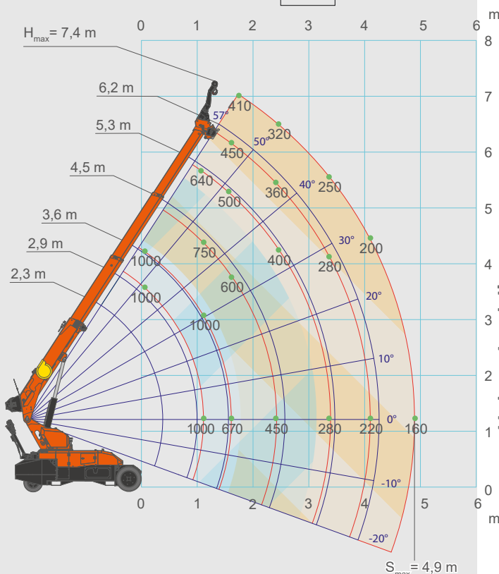
Säulenschwenkhaken-Lastdiagramm
