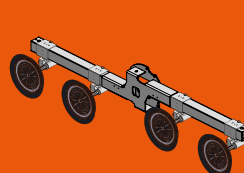
Ø290 en ligne
