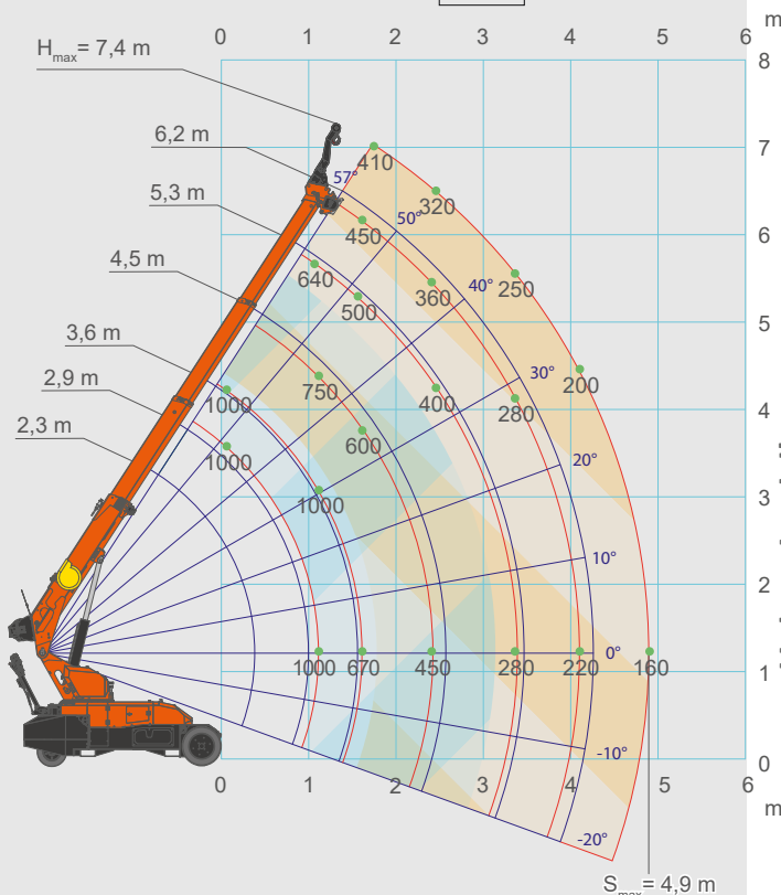
Säulenschwenkhaken-Lastdiagramm
