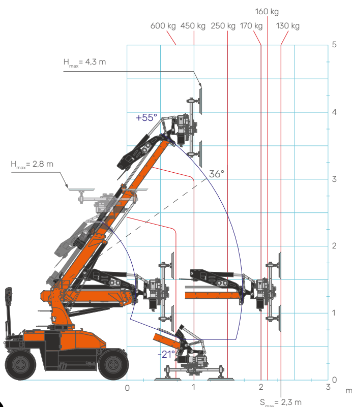
Manipulator-Lastdiagramm
