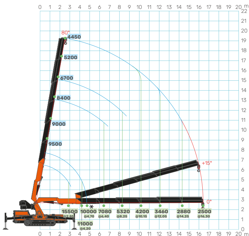
Braccio principale
