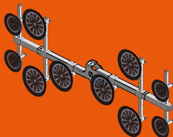
Ø400 - 10 Sauger
