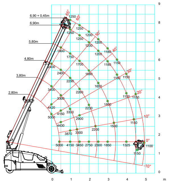
Haken-Lastdiagramm
