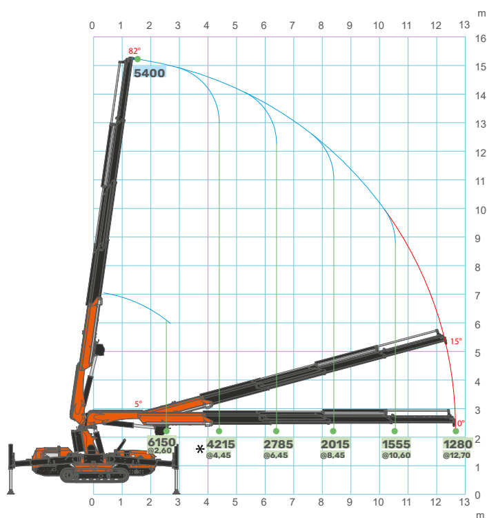
Braccio principale
